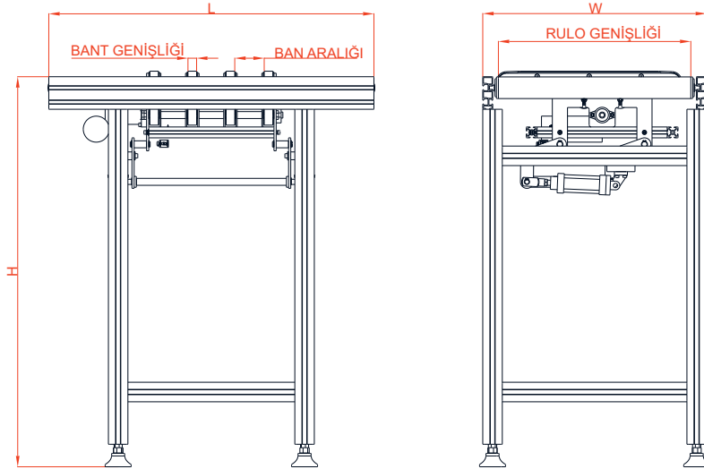
STANDART AKTARMA KONVEYÖR ÖLÇÜLERİ STANDARD TRANSFER CONVEYOR DIMENSIONS
