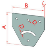
Dereceli T Bağlantı Sacı Kod: 3.003.23127.03
