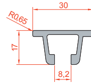
Yan Bariyer Profili (40) Kod: 1.2.00.017040.00
