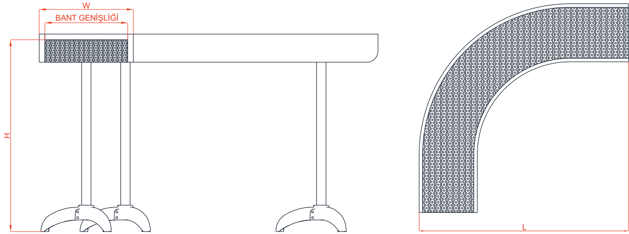
STANDART MODÜLER BANTLI KONVEYÖR ÖLÇÜLERİ STANDARD MODULAR BELT CONVEYOR DIMENSIONS
