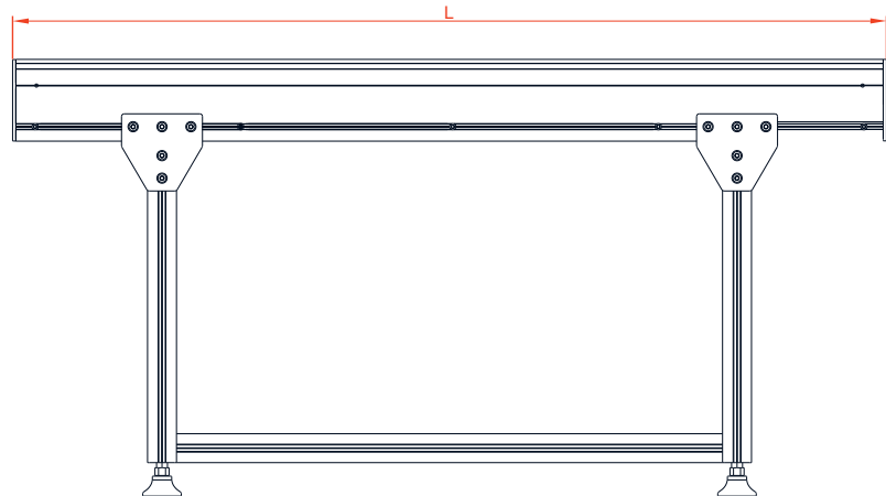
STANDART AVARE RULOLU KONVEYÖR ÖLÇÜLERİ STANDARD HALL ROLLER CONVEYOR DIMENSIONS
