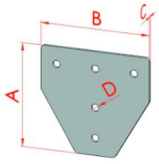
T Bağlantı Sacı Kod: 3.003.23127.01
