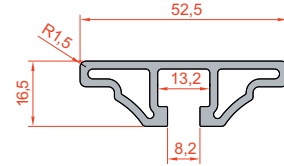
Yan Bariyer Profili (60) Kod: 1.2.00.016060.00
