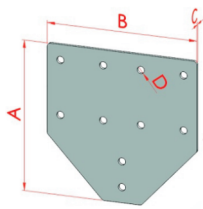
Ek T Bağlantı Sacı Kod: 3.003.23127.02
