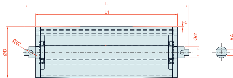
Ø114 Gergi Tamburu
