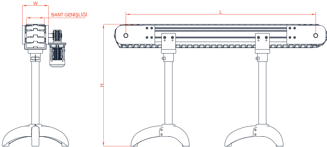
STANDART ASETAL BANTLI KONVEYÖR ÖLÇÜLERİ STANDARD ACETAL BELT CONVEYOR DIMENSIONS
