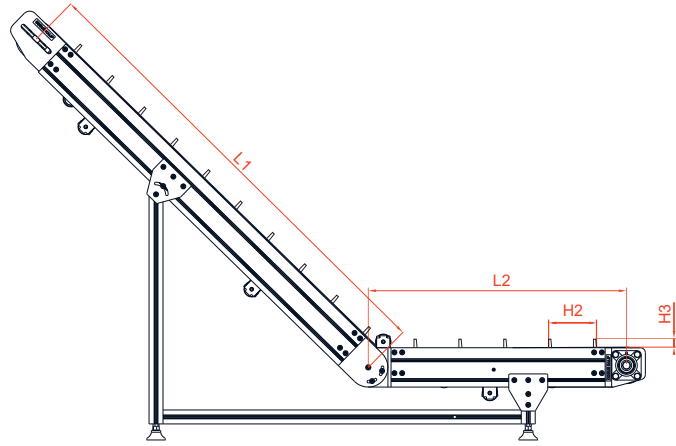
STANDART (L) ELEVATÖR KONVEYÖR ÖLÇÜLERİ STANDARD (L) ELEVATOR CONVEYOR SIZES
