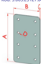
Düz Ek Bağlantı Sacı Kod: 3.003.23075.04 Kod: 3.003.23127.04
