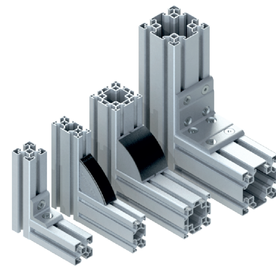
Fixations et Accessoires
