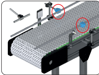
Sabot de guidage Porte-croix
