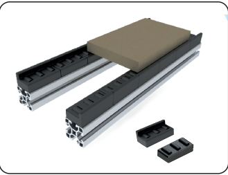
Roulement retour inférieur
